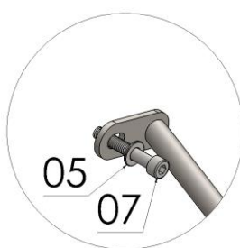
Detalhe B
