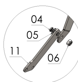
Detalhe D
