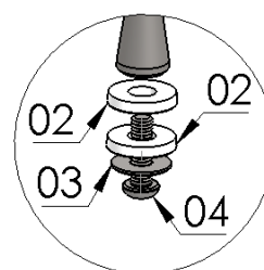
DETALHE A1 ESCALA 2 : 5
