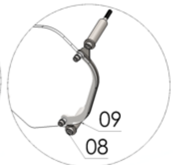
Detalhe D
