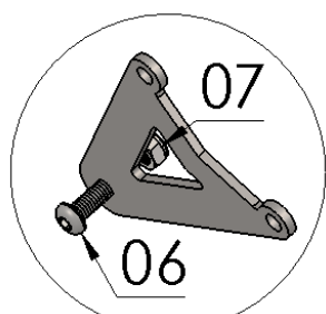
DETALHE D1 ESCALA 2 : 5
