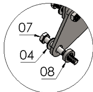
DETALHE A1 ESCALA 2 : 5
