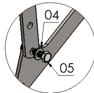
DETALHE C1 ESCALA 2 : 5
